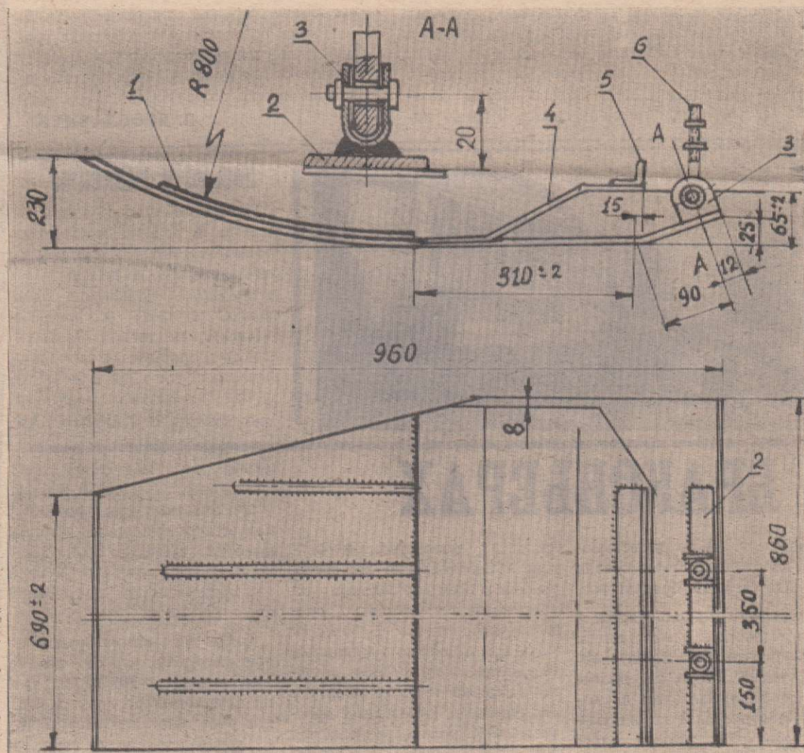
Рис. 1. Приспособление к жатке ЖВН-6 для сдвигания валков: 1 — щиток, 2 — полоса, 3 — скоба, 4 — козырек, 5 — угольник, 6 — специальный болт.
