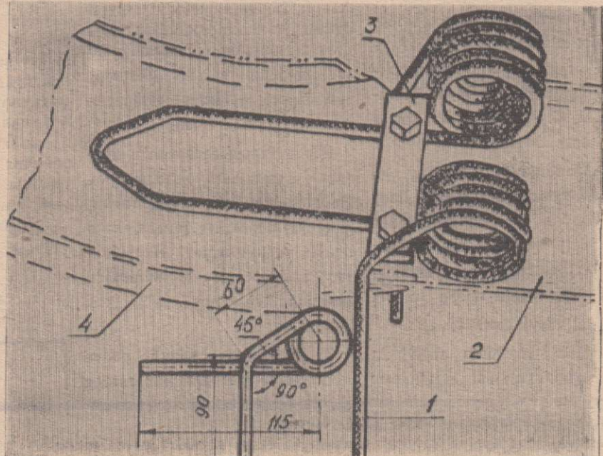
Рис. 1. Приспособление к жатке ЖВН-6 для сдвигания валков: 1 — щиток, 2 — полоса, 3 — скоба, 4 — козырек, 5 — угольник, 6 — специальный болт.
